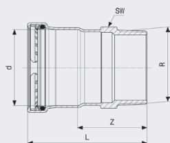
Profipress G XL-přechodový kus - měď model 2611XL
