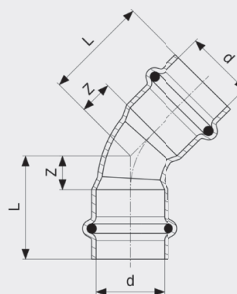
Profipress G-oblouk 45° - měď model 2626
