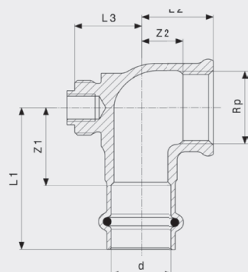
Profipress G-připojovací koleno 90° - červený bronz model 2614.6
