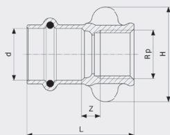
Profipress G-přechodový kus - červený bronz model 2612.3
