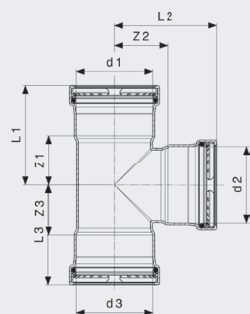
Profipress G XL-T-kus - měď model 2618XL
