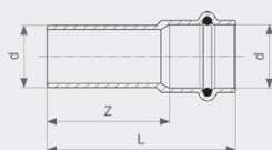
Profipress G-přechodový kus - červený bronz model 2613
