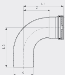
Profipress G XL-oblouk 90° - měď model 2616.1XL
