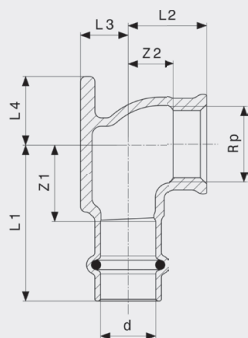
Profipress G-nástěnka - červený bronz model 2625.5
