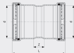
Profipress G XL-objímka - měď model 2615XL
