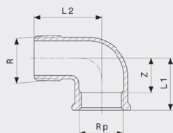
Připojovací koleno 90° - červený bronz model 2614.5
