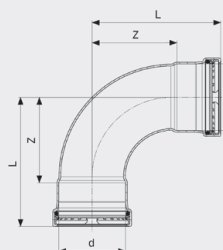
Profipress G XL-oblouk 90° - měď model 2616XL
