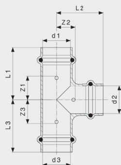
Profipress G-T-kus - měď model 2618
