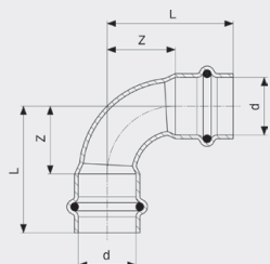
Profipress G-oblouk 90° - měď model 2616
