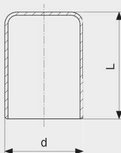
Profipress-zátka - měď model 2457
