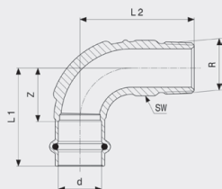
Profipress G-přechodový oblouk 90° - červený bronz model 2614
