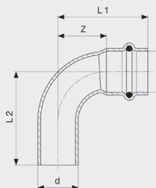
Profipress G-oblouk 90° - měď model 2616.1
