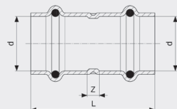
Profipress G-objímka - měď model 2615
