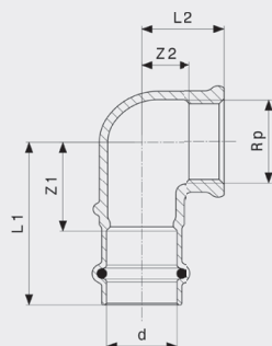
Profipress G-přechodové koleno 90° - červený bronz model 2614.2
