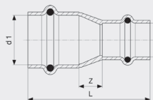
Profipress G-redukční objímka - měď model 2615.2
