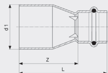
Profipress G-redukce - měď model 2615.1
