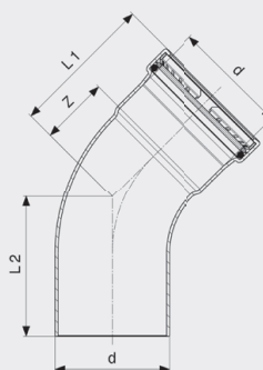
Profipress G XL-oblouk 45° - měď model 2626.1XL
