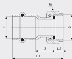
Profipress G-připojovací šroubení - červený bronz model 2666
