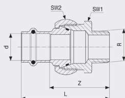
Profipress G-přechodové šroubení - červený bronz model 2654
