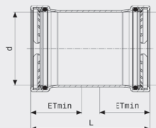
Profipress G XL-posuvná objímka - měď model 2615.5XL
