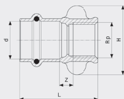
Profipress G-přechodový kus - červený bronz model 2612
