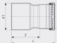
Profipress G XL-redukce - měď model 2615.1XL
