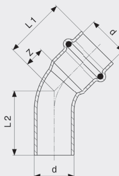
Profipress G-oblouk 45° - měď model 2626.1
