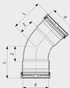
Profipress G XL-oblouk 45° - měď model 2626XL
