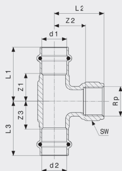
Profipress G-T-kus - červený bronz model 2617.2
