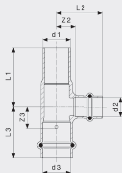
Profipress G-T-kus - měď model 2618.1
