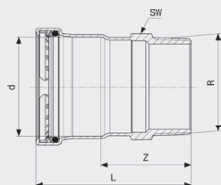
Profipress G-přechodový kus - červený bronz model 2611
