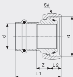
Profipress G-připojovací šroubení - červený bronz model 2661
