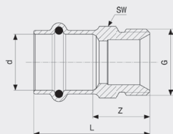
Profipress G-přechodový kus - červený bronz model 2611.5
