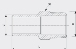
Sanpress-zásuvný kus - červený nebo křemíkový bronz model 2211.1
