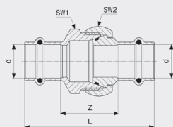
Profipress G-šroubení - červený bronz model 2650
