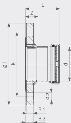
Profipress G XL-přírubový přechod - měď model 2659.5XL
