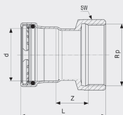
Profipress G XL-přechodový kus - měď model 2612XL
